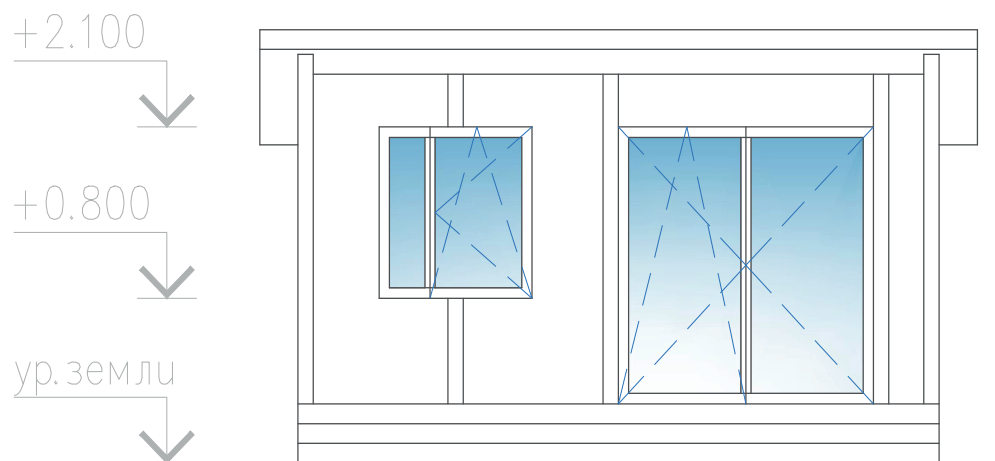
Фасада 1-3
