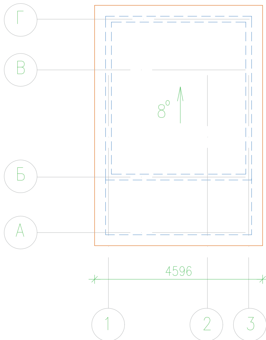
План кровли
