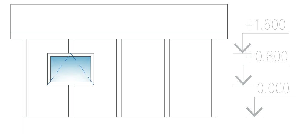
Фасада 3-1
