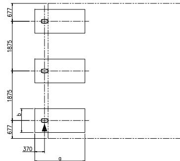
柱・基礎位置図 (S = 1/50) ▶: 排水位置を示す
