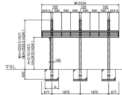
側面図 (S = 1/50)
