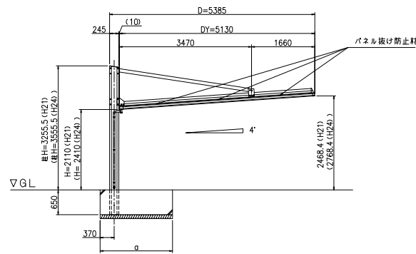
正面図 (S = 1/50)
