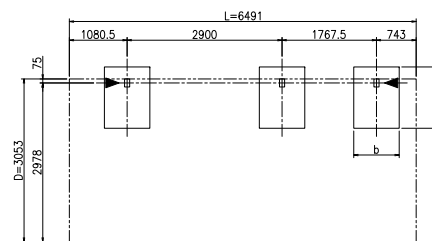
柱・基礎位置図 (S = 1 / 50) ▶ : 排水位置を示す
