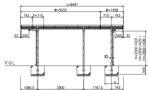
立面図 (S = 1 / 50)
