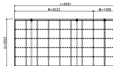
平面図 (S = 1 / 50)
