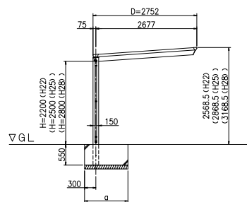
正面図 (S = 1 / 50)
