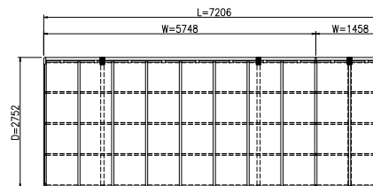
平面図 (S = 1 / 50)
