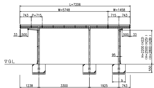
立面図 (S = 1 / 50)
