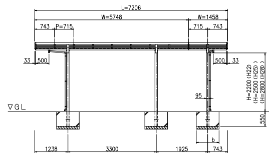
立面図 (S = 1 / 50)
