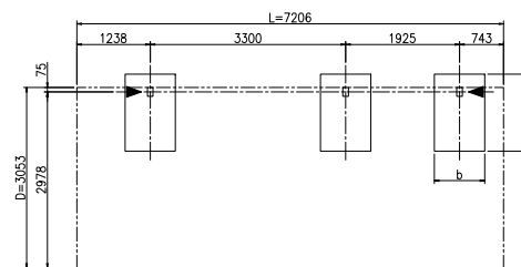
柱・基礎位置図 (S = 1 / 50) ▶ : 排水位置を示す
