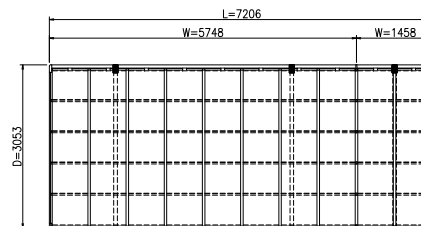
平面図 (S = 1 / 50)
