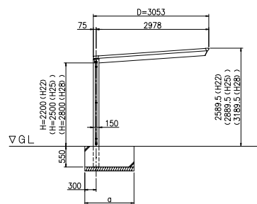
正面図 (S = 1 / 50)
