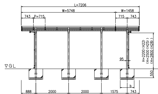
立面図 (S = 1 / 50)
