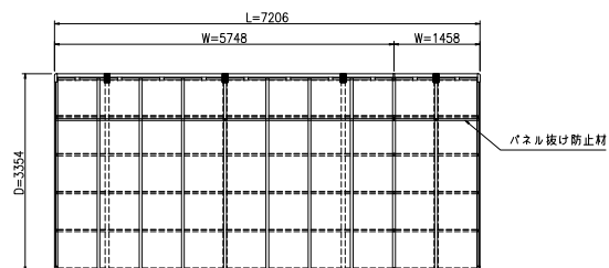
平面図 (S = 1 / 50)
