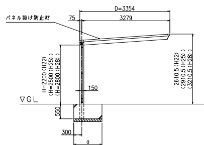
正面図 (S = 1 / 50)
