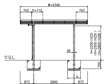
立面図 (S = 1 / 50)
