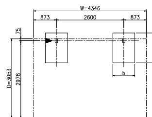
柱・基礎位置図 (S = 1 / 50) ▶ : 排水位置を示す
