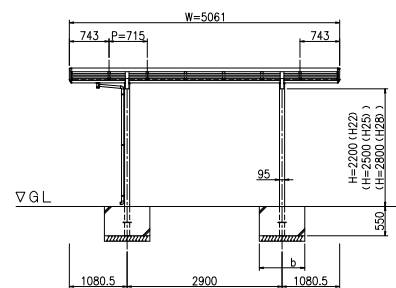
立面図 (S = 1 / 50)
