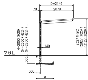
正面図 (S = 1 / 50)
