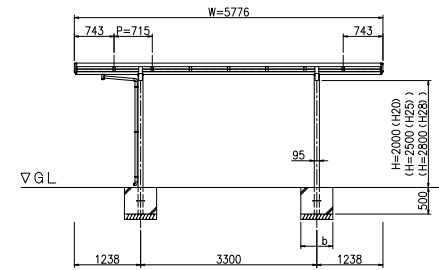
立面図 (S = 1 / 50)
