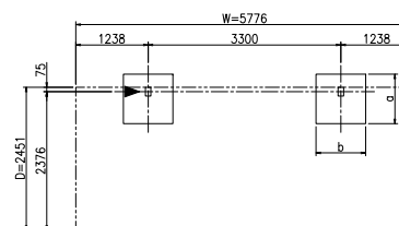
柱・基礎位置図 (S = 1 / 50) ▶: 排水位置を示す
