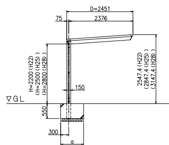
正面図 (S = 1 / 50)
