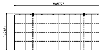
平面図 (S = 1 / 50)
