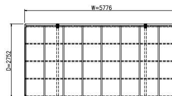
平面図 (S = 1 / 50)
