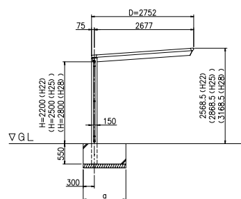
正面図 (S = 1 / 50)
