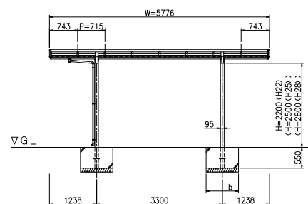
立面図 (S = 1 / 50)
