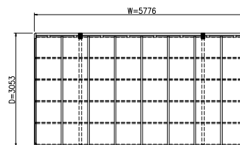
平面図 (S = 1/50)
