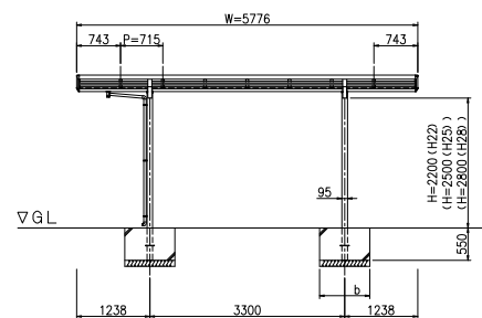
立面図 (S = 1/50)
