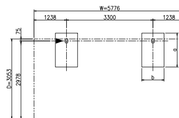
柱・基礎位置図 (S = 1/50) ▶ : 排水位置を示す
