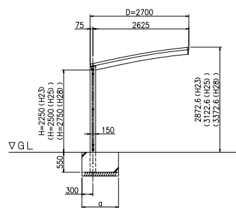
正面図 (S = 1 / 50)
