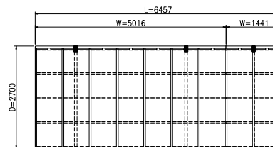
平面図 (S = 1 / 50)
