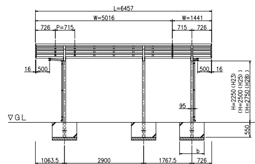
立面図 (S = 1 / 50)
