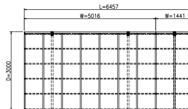
平面図 (S = 1 / 50)
