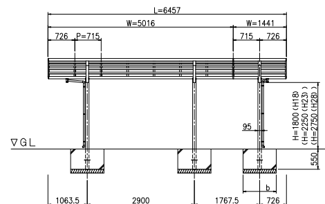
立面図 (S = 1 / 50)
