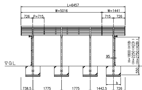
立面図 (S = 1 / 50)
