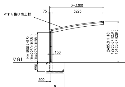
正面図 (S = 1 / 50)
