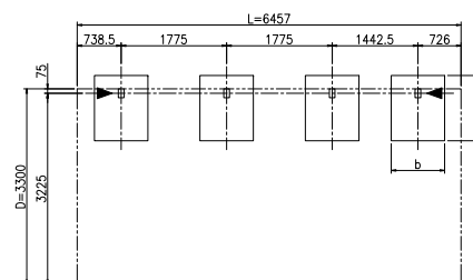
柱・基礎位置図 (S = 1 / 50) ▶: 排水位置を示す
