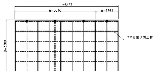
平面図 (S = 1 / 50)
