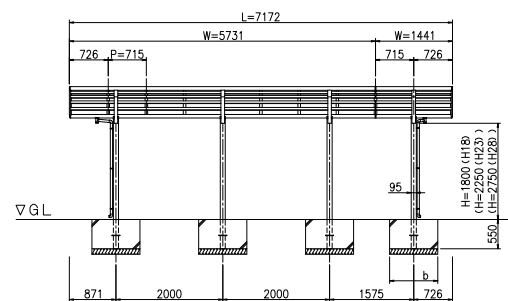
立面図 (S = 1 / 50)
