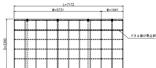
平面図 (S = 1 / 50)
