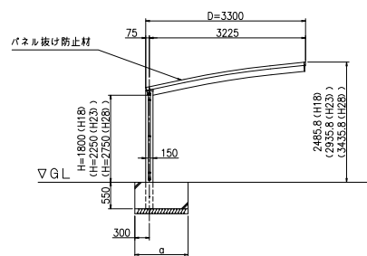
正面図 (S = 1 / 50)
