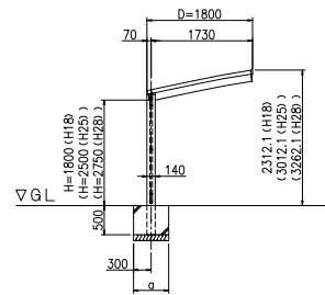
正面図 (S = 1 / 50)
