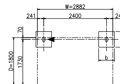
柱・基礎位置図 (S = 1 / 50)
