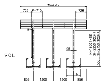
立面図 (S = 1/50)
