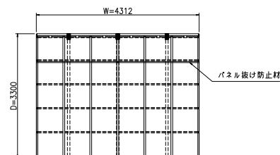
平面図 (S = 1/50)
