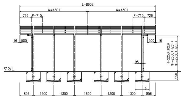
立面図 (S = 1 / 50)
