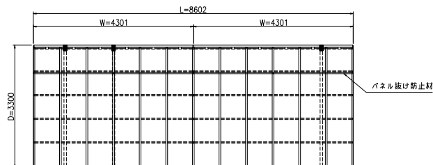
平面図 (S = 1 / 50)
