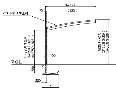
正面図 (S = 1 / 50)
