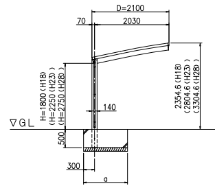
正面図 (S=1/50)
