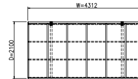
平面図 (S=1/50)
