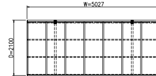
平面図 (S = 1 / 50)
