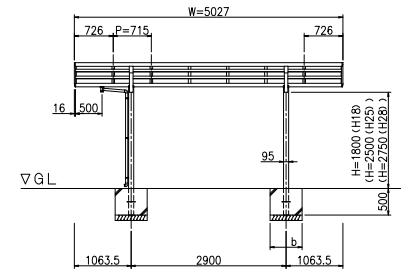
立面図 (S = 1 / 50)
