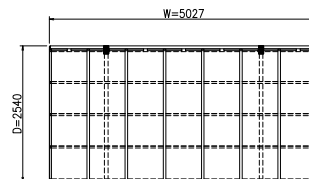
平面図 (S = 1 / 50)
