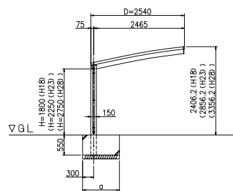
正面図 (S = 1 / 50)
