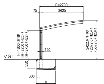
正面図 (S = 1 / 50)
