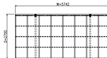
平面図 (S = 1 / 50)
