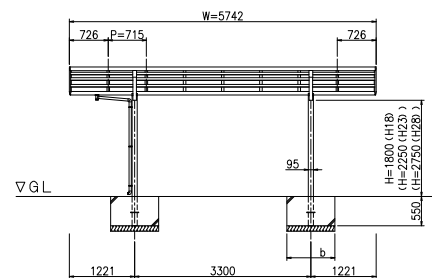
立面図 (S = 1 / 50)
