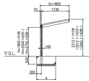
正面図 (S = 1 / 50)
