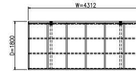
平面図 (S = 1 / 50)
