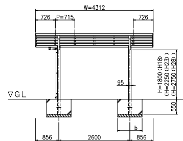
立面図 (S = 1 / 50)
