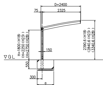
正面図 (S = 1 / 50)
