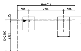
柱・基礎位置図 (S = 1 / 50) ▶ : 排水位置を示す
