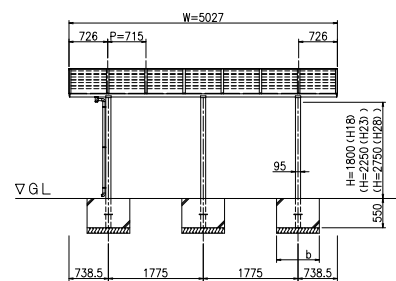
立面図 (S = 1/50)
