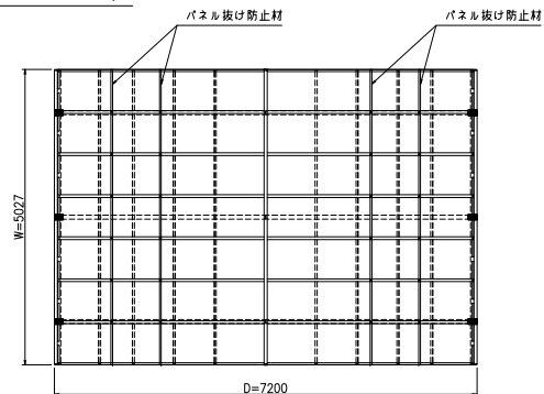
平面図 (S = 1/50)
