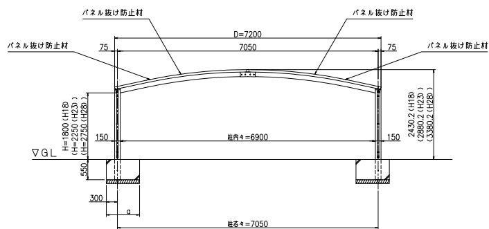
正面図 (S = 1/50)
