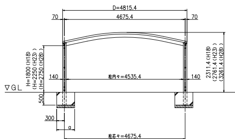
正面図 (S = 1 / 50)
