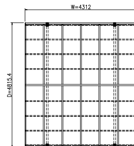
平面図 (S = 1 / 50)
