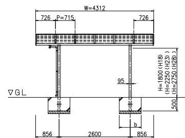
立面図 (S = 1 / 50)
