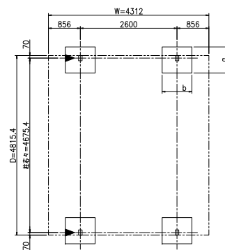
柱・基礎位置図 (S = 1 / 50)
