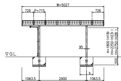
立面図 (S = 1 / 50)
