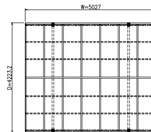
平面図 (S = 1 / 50)
