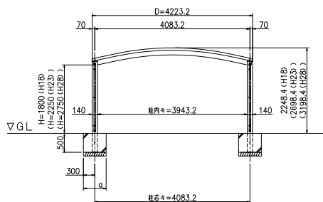
正面図 (S = 1 / 50)
