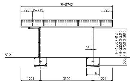
立面図 (S = 1 / 50)
