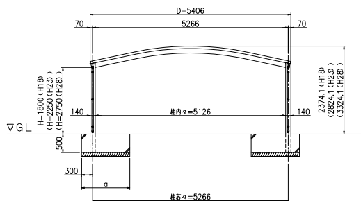
正面図 (S = 1 / 50)
