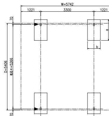
柱・基礎位置図 (S = 1 / 50) ▶: 排水位置を示す
