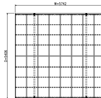
平面図 (S = 1 / 50)
