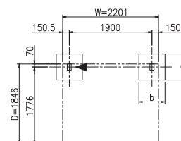
ZÁKLADY - SLOUPY (S = 1 / 50)
