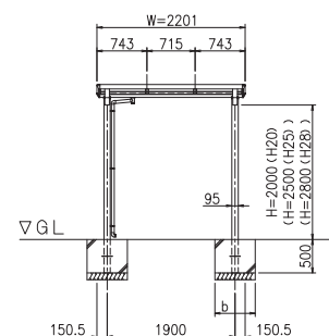
ŘEZ (S = 1 / 50)
