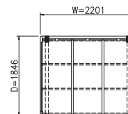
PŮDORYS (S = 1 / 50)
