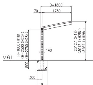
ČELNÍ POHLED (S = 1 / 50)
