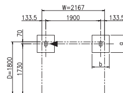
ZÁKLADY - SLOUPY (S = 1 / 50)
