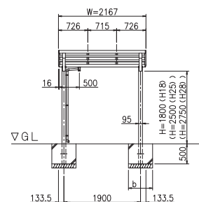
ŘEZ (S = 1 / 50)
