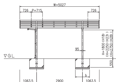
ŘEZ (S = 1 / 5 0)
