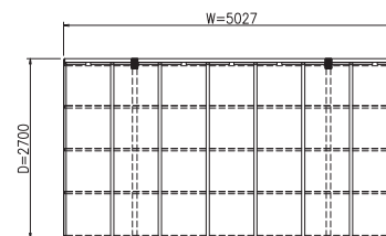
PŮDORYS (S = 1 / 5 0)
