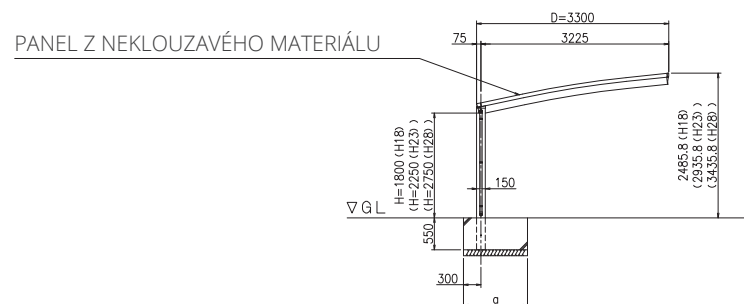
ČELNÍ POHLED (S = 1 / 5 0)
