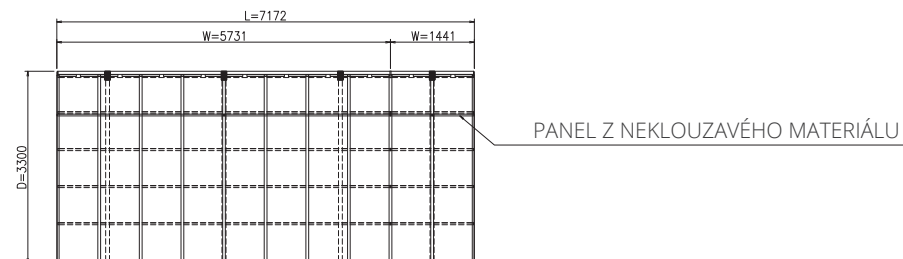
PŮDORYS (S = 1 / 5 0)
