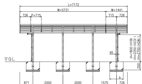
ŘEZ (S = 1 / 5 0)
