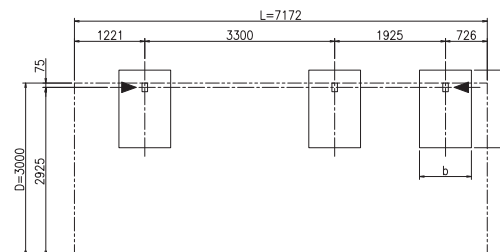
ZÁKLADY - SLOUPY (S = 1 / 50) ► ODTOKY / OKAPY
