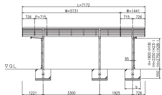
ŘEZ (S = 1 / 50)
