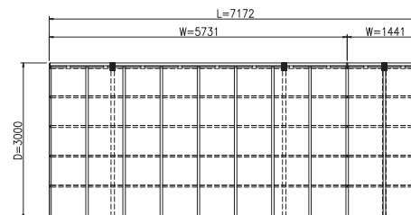
PŮDORYS (S = 1 / 50)
