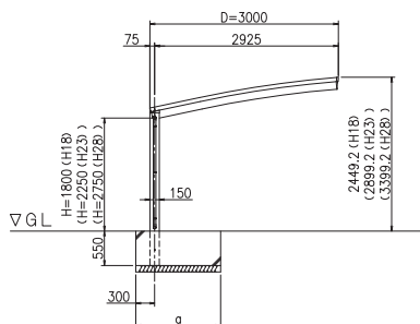
ČELNÍ POHLED (S = 1 / 50)
