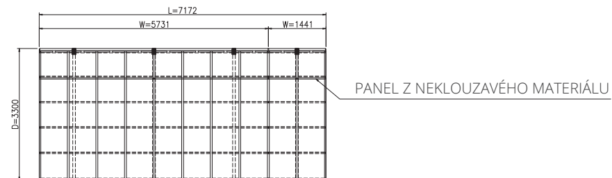
PŮDORYS (S = 1 / 50)
