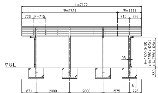
ŘEZ (S = 1 / 50)
