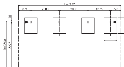
ZÁKLADY - SLOUPY (S = 1 / 50) ► ODTOKY / OKAPY
