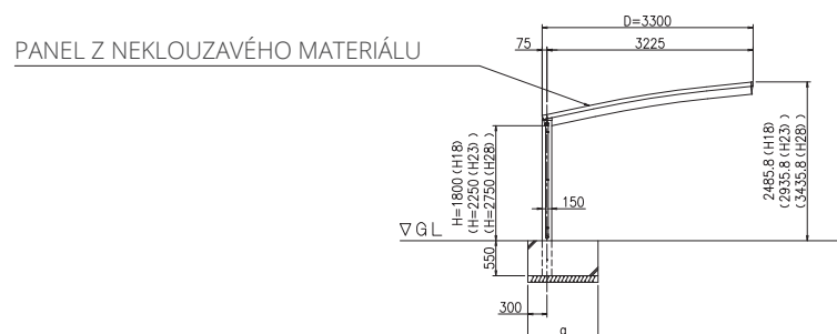
ČELNÍ POHLED (S = 1 / 50)
