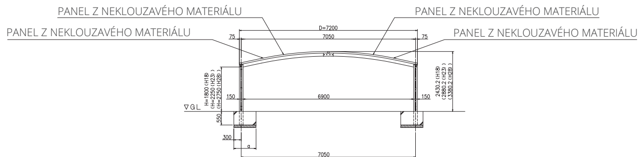
ČELNÍ POHLED (S = 1 / 5 0)
