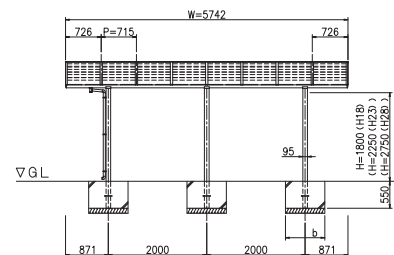
ŘEZ (S = 1 / 5 0)
