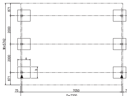
ZÁKLADY - SLOUPY (S = 1 / 5 0) ▶ ODTOKY / OKAPY
