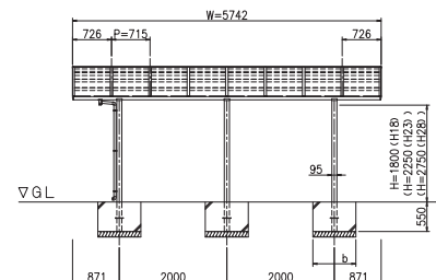
ŘEZ (S = 1 / 50)
