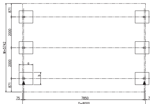
ZÁKLADY - SLOUPY (S = 1 / 50) ▶ ODTOKY / OKAPY
