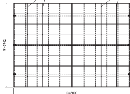
PŮDORYS (S = 1 / 50) PANEL Z NEKLOUZAVÉHO MATERIÁLU
