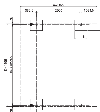
ZÁKLADY - SLOUPY (S = 1 / 50) ▶ ODTOKY / OKAPY
