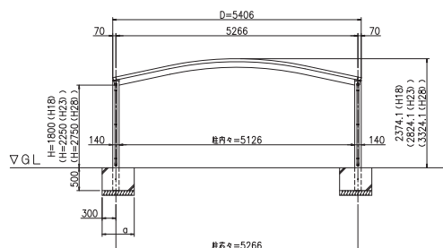
ČELNÍ POHLED (S = 1 / 50)
