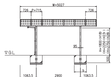
ŘEZ (S = 1 / 50)
