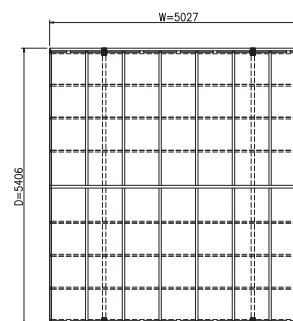
PŮDORYS (S = 1 / 50)
