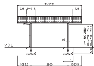
ŘEZ (S = 1 / 50)
