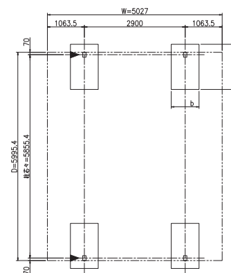
ZÁKLADY - SLOUPY (S = 1 / 50) ▶ ODTOKY / OKAPY
