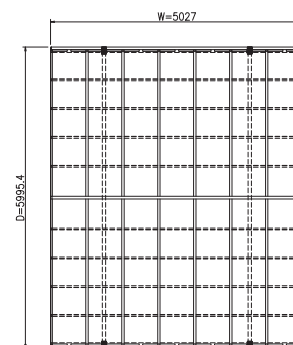
PŮDORYS (S = 1 / 50)
