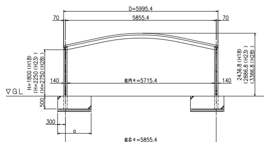
ČELNÍ POHLED (S = 1 / 50)
