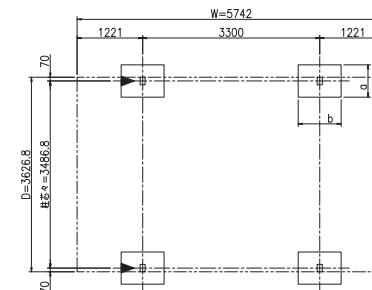
ZÁKLADY - SLOUPY (S = 1 / 50) ▶ ODTOKY / OKAPY
