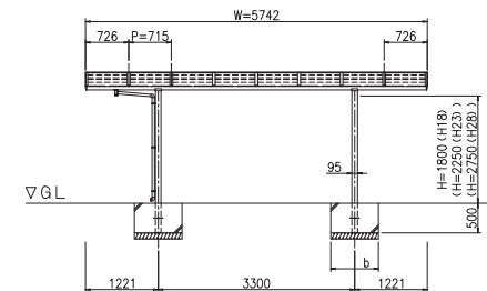
ZÁKLADY - SLOUPY (S = 1 / 50) ▶ ODTOKY / OKAPY
