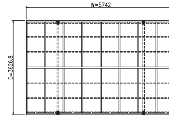
PŮDORYS (S = 1 / 50)
