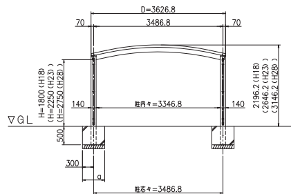
ČELNÍ POHLED (S = 1 / 50)
