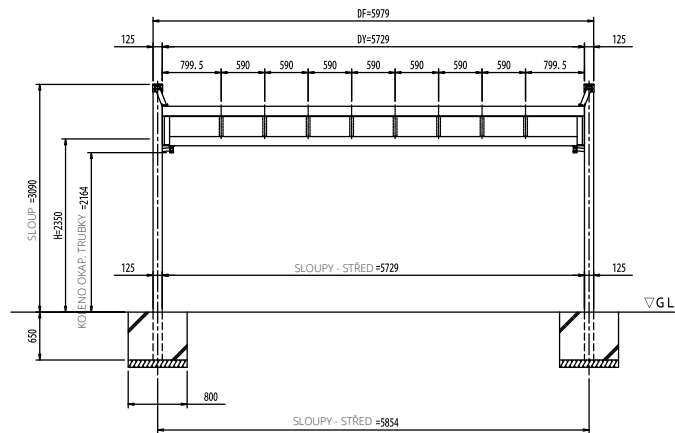
ŘEZ (S=1/50)
