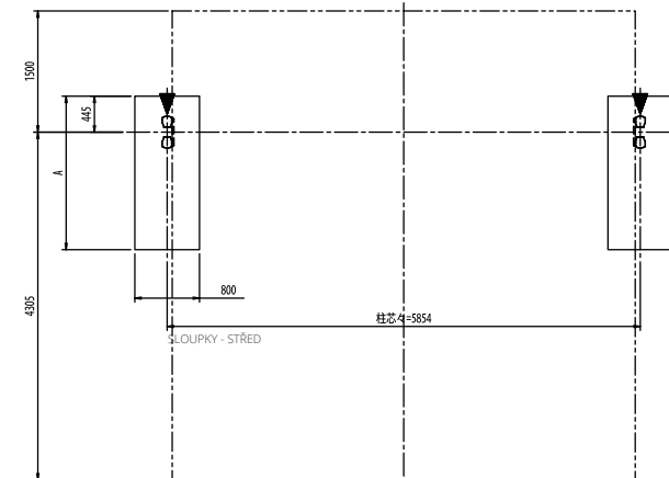
PŮDORYS ZÁKLADŮ (S=1/50)
