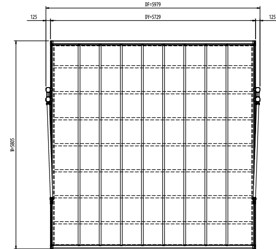
PŮDORYS ZÁKLADŮ (S=1/50)
