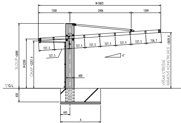
BOČNÍ POHLED (S=1/50)
